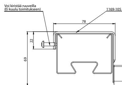
AMRPK päätykannatin korkealla kiinnikkeellä (tilattava erikseen).
