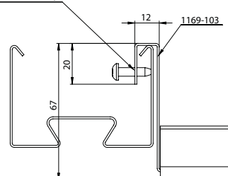
AMRPK päätykannatin ja laskeva kiinnike ruuvi- tai puristuslukituksella (tilattava erikseen).
