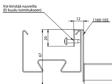
AMRPK päätykannatin ja laskeva kiinnike ruuvi- tai puristuslukituksella (tilattava erikseen).
