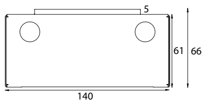
Pääty (LED-mallit ilman murtoaihoita)
