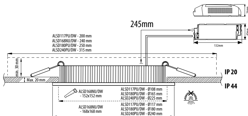
Velox-paneelin mitoitus uppoasennuksessa
