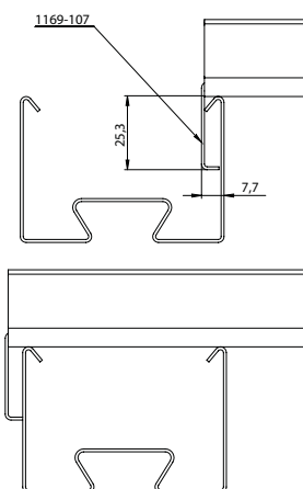
AMRPK päätykannatin vakiokiinnikkeellä.
