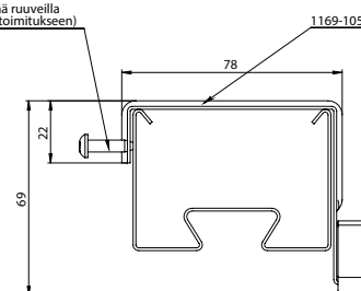
AMRPK päätykannatin korkealla kiinnikkeellä (tilattava erikseen).
