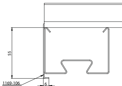
AMRPK päätykannatin ja laskeva kiinnike ruuvi- tai puristuslukituksella (tilattava erikseen). Laskevan kiinnikkeen avulla saadaan ramppivalaisin samalle tasolle kuin ripustuskiskoon AMJK2-kiinnikkeellä asennetut valaisimet.
